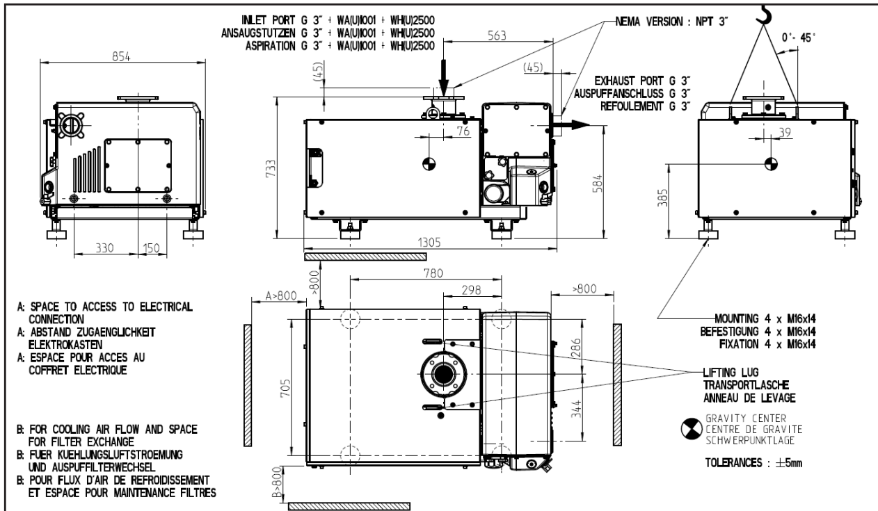
SV 470 BF /SV570 BF 尺寸图
