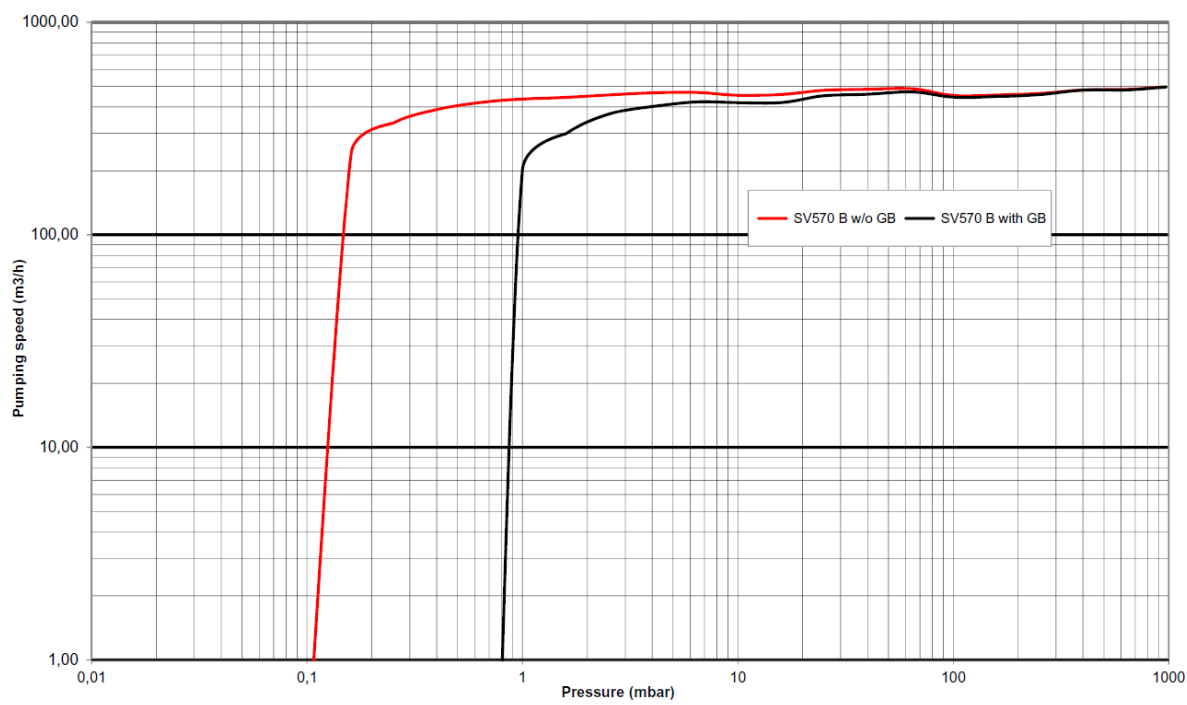
SV 570B 抽速曲线
